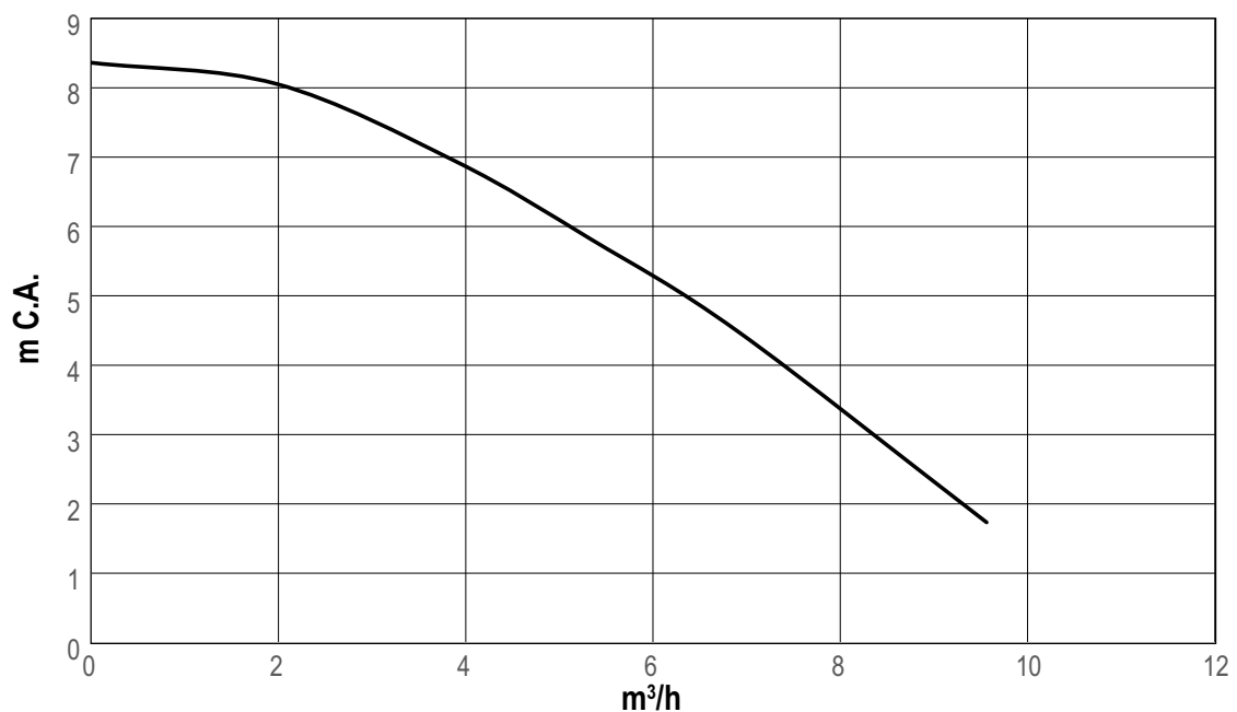
fig. 118 - Diagramma prevalenza
