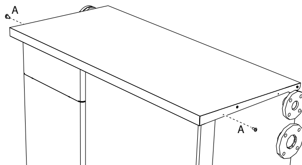
fig. 103 - Apertura coperchio
